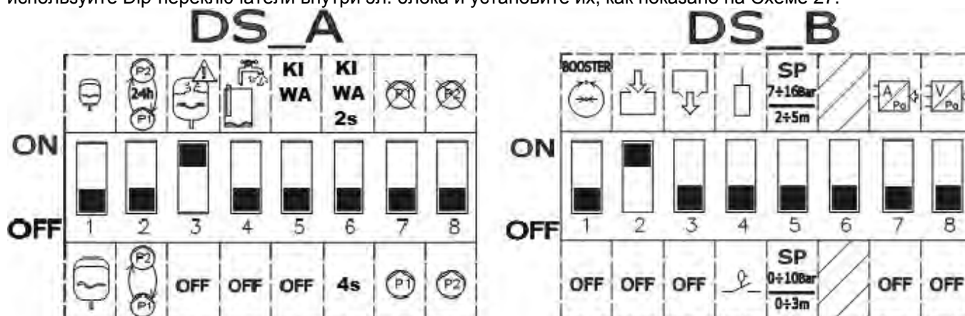
Схема 27: Настройка Dip-переключателей заполнения
